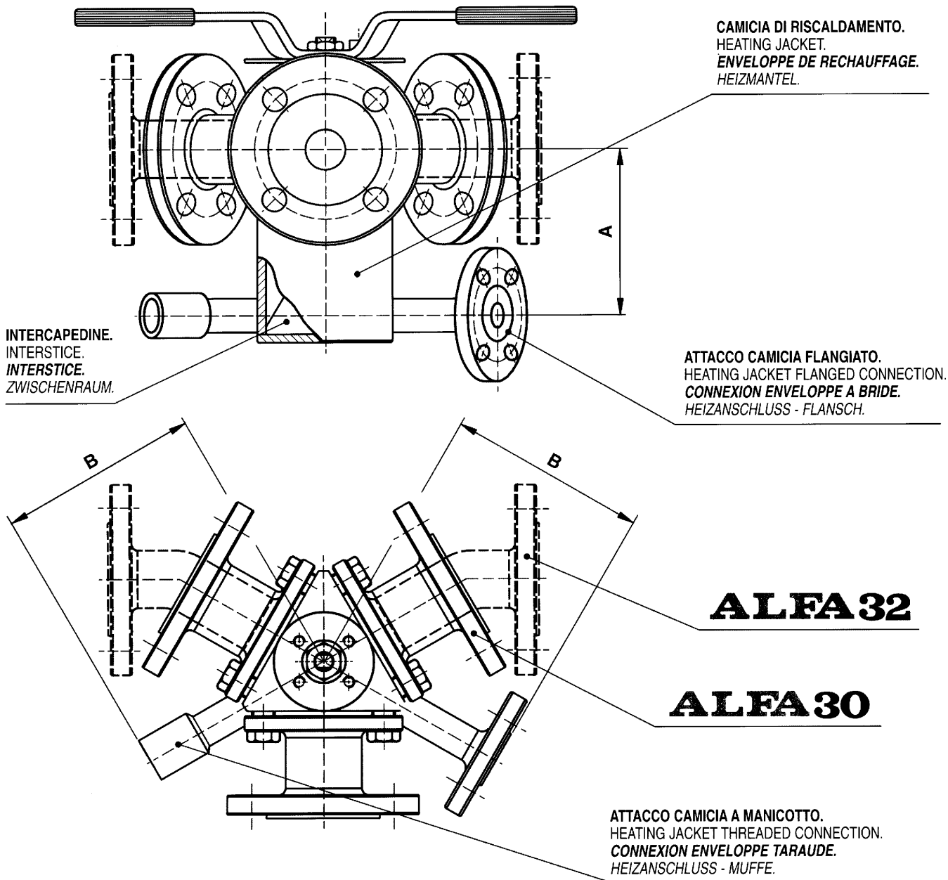
DIMENSIONI - DIMENSIONS - DIMENSIONS - ABMESSUNGEN
